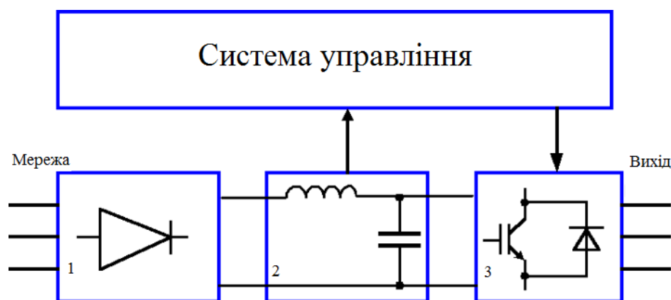
Рис.1. Структурна схема конвертера
